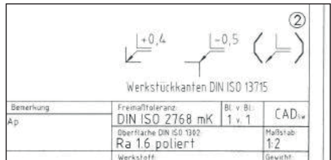
Bemaßungsbeispiel
