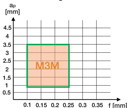
DCMT 13T508-M3M-SL Anwendungsbereich
