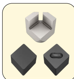
CNGN 1207 / CNGX 1207
