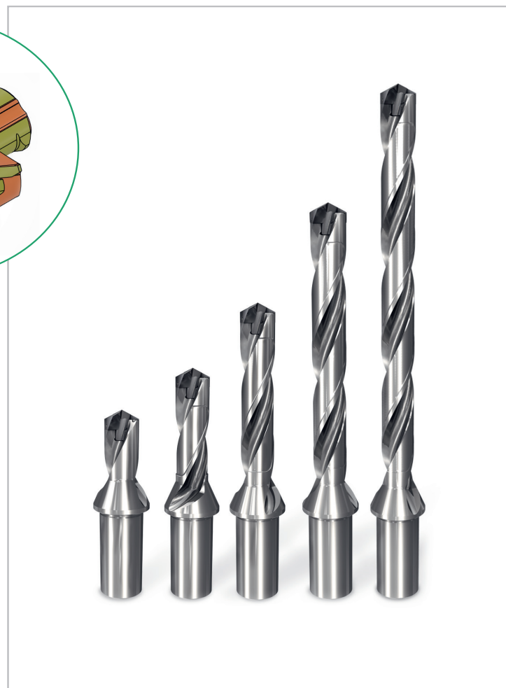
ISCARs SUMOCHAM-System bietet im Standard Bohrer mit Wechselköpfen in Durchmessern von vier bis 32,9 Millimetern und in Längen von 1,5 bis 12xD.
