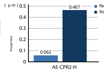
Oberflächenrauigkeit
