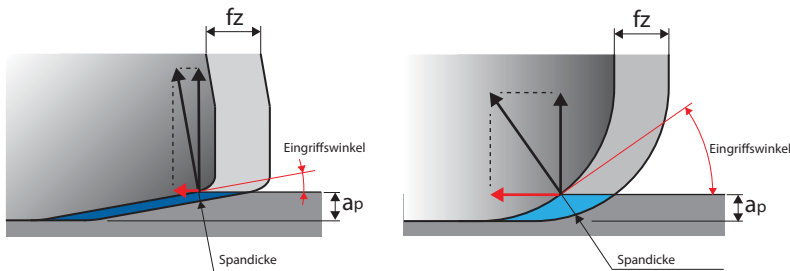
Radienübergänge
